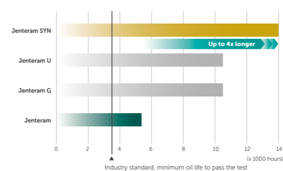
Oxidation Stability Test Results/Výsledky testu oxidační stability (test method TOST ASTM D943) / (testovací metoda TOST ASTM D943)
