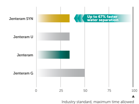
Water Separability Test Results/Výsledky testu oddělitelnosti vody (test method ASTM D1401) / (testovací metoda ASTM D1401)
