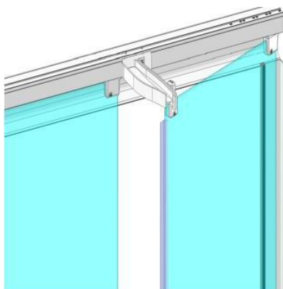
Detail horní výjezd
