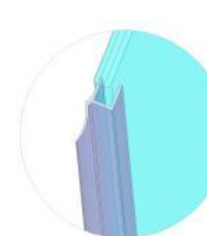
DETAIL MEZISKLENÍHO TĚSNĚNÍ
